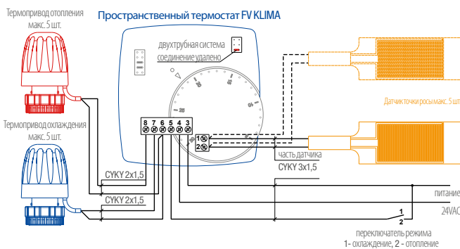
Двухтрубная система - схема подключения
