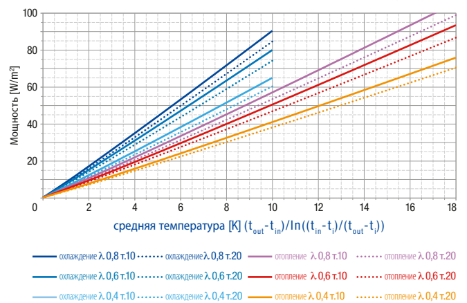
Охлаждающий мат CoolGRID с расстоянием 29 мм под разной штукатуркой
