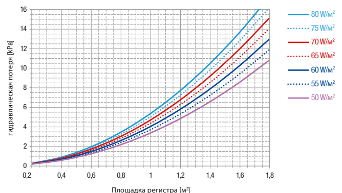
Гидравлическая потеря регистра, расстояние 40 мм, \Delta T 3 К
