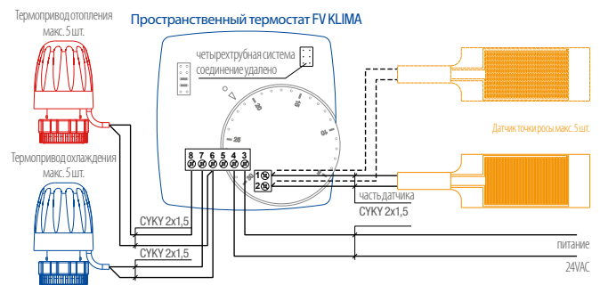
Четырехтрубная система - схема подключения
