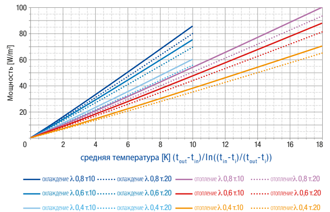
Охлаждающий мат CoolGRID с расстоянием 50 мм под разной штукатуркой
