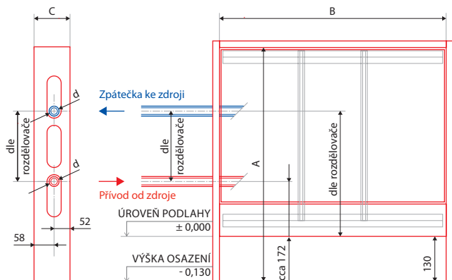
Obr. č. 20: Napojení přívodu a zpátečky z boku - horizontálně do skříň pod omítku
